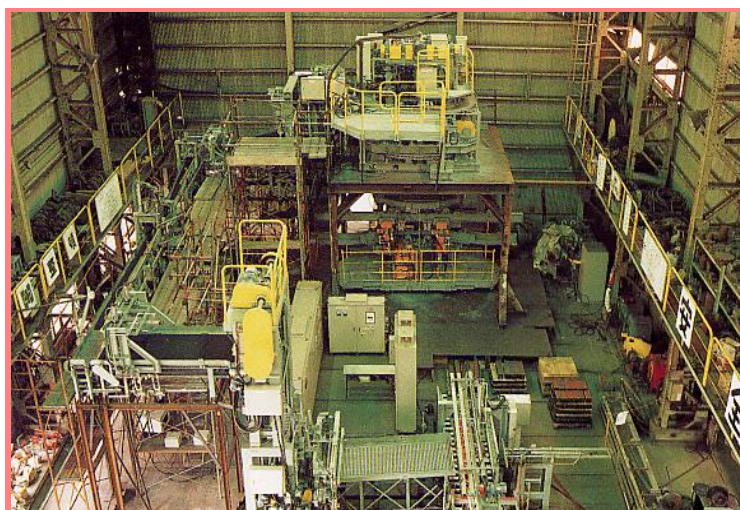
省力化設備組立・試運転
