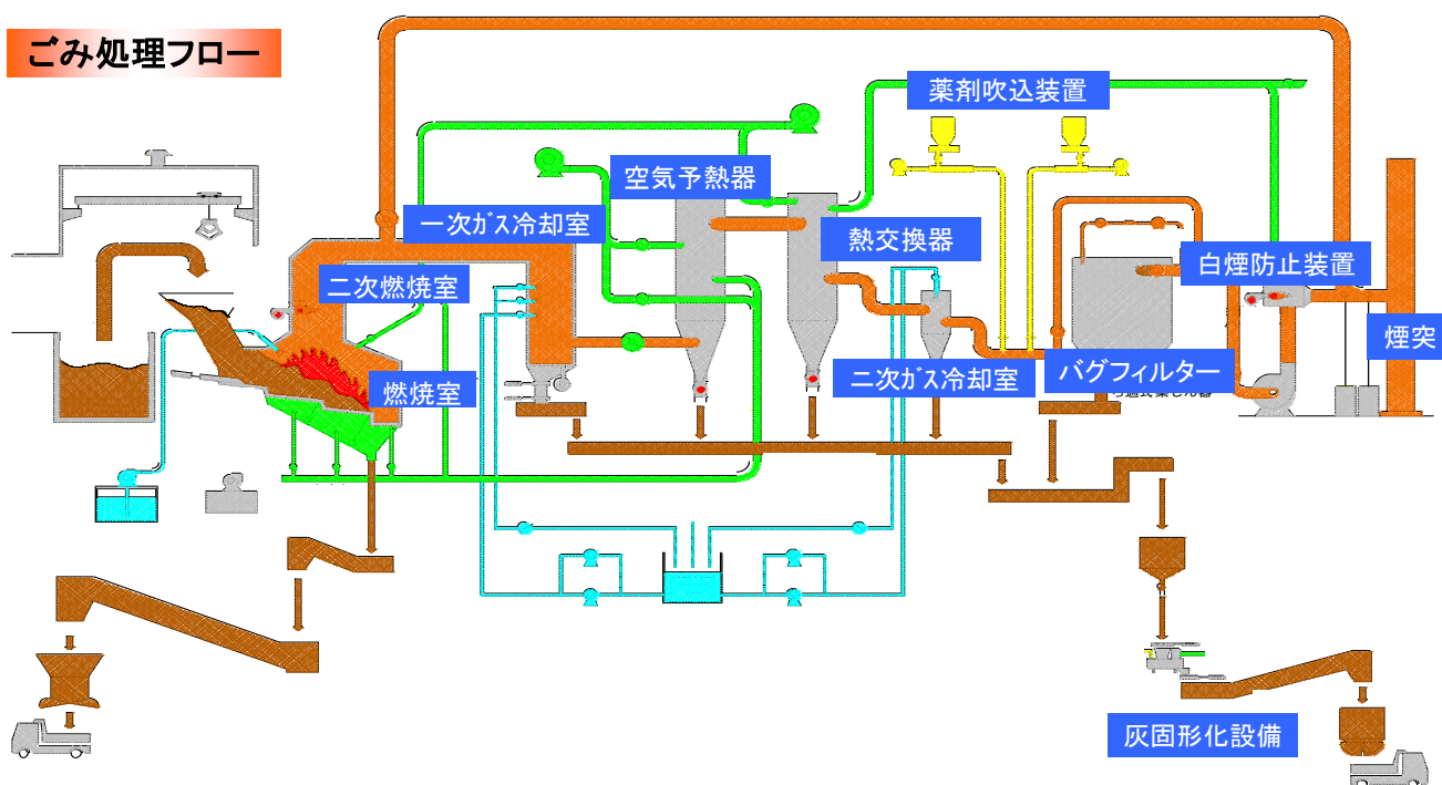
都市ごみ焼却施設
