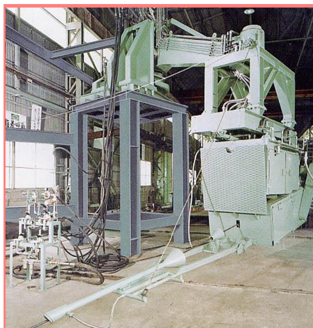
高炉出銑口酸素開孔機
