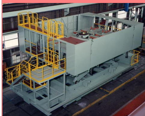
炉底分離式転炉築炉設備
